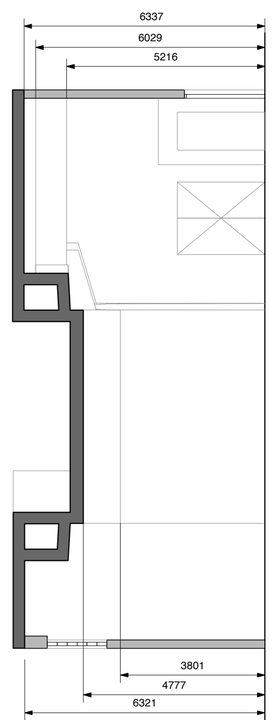
dwarsdoosnede BB'
