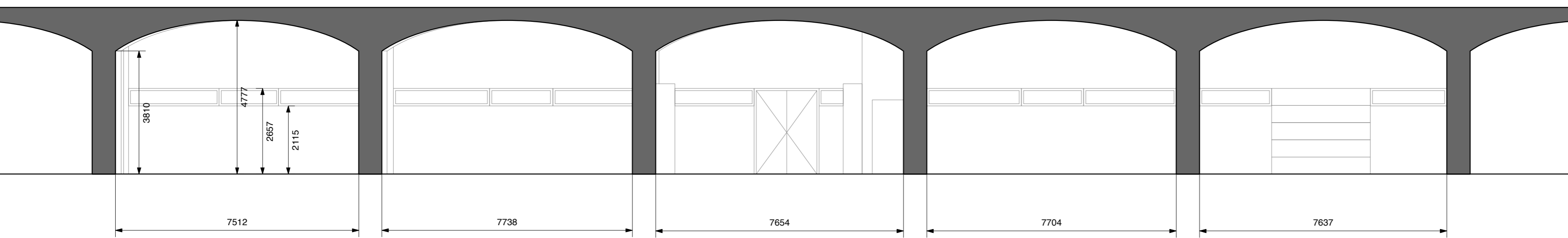
langsdoosnede AA'
